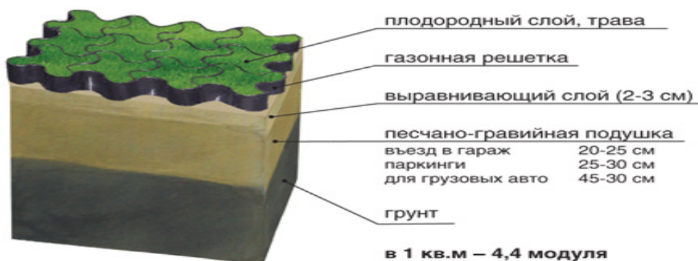
Схема устройства экопарковки
